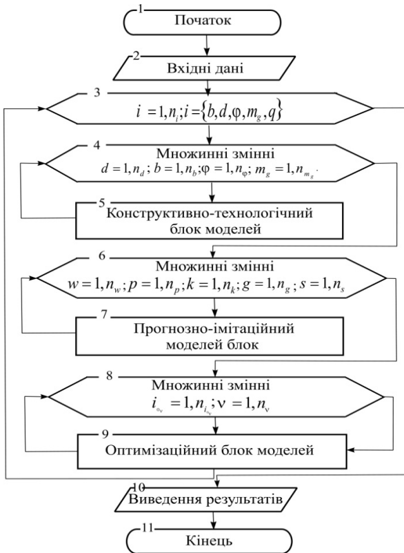
Рисунок 1. Блок-схема оптимізаційних розрахунків з обґрунтування оптимальних конструкцій та параметрів меліоративних систем
